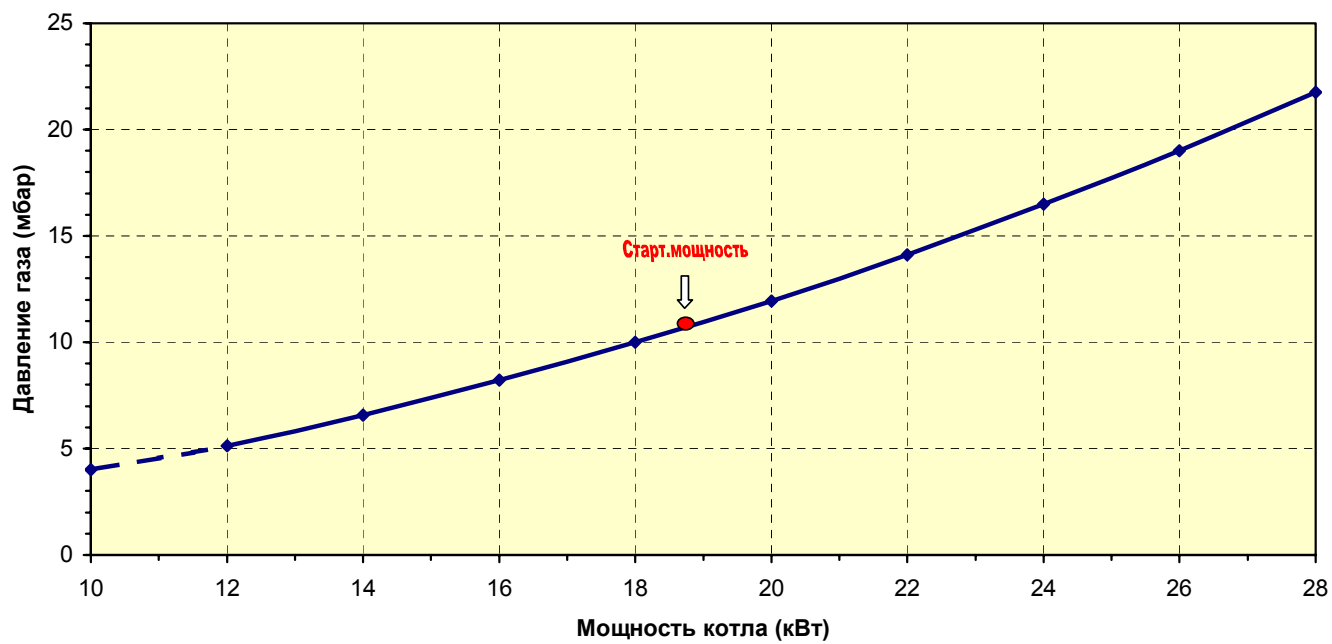
График настройки мощности THERM 28 (пропан), форсунки - 0.82 мм
