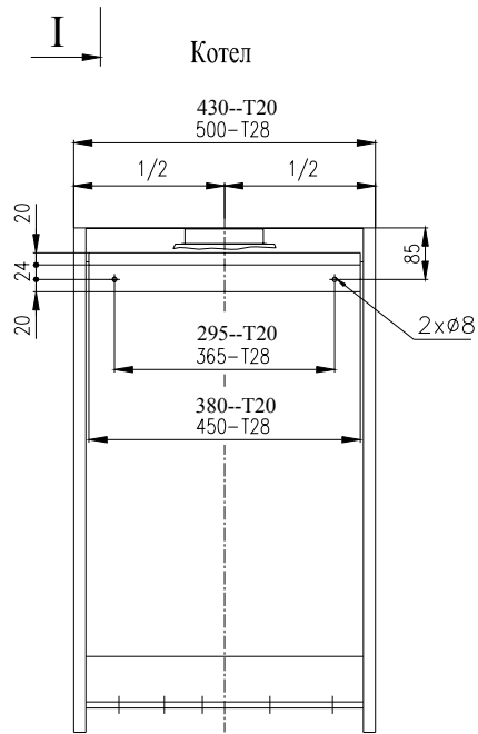
I | Разрез по I-I
