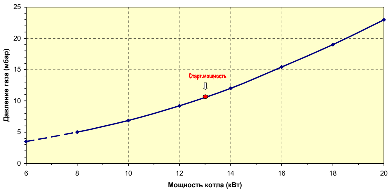
График настройки мощности THERM 20 (пропан), форсунки - 0.82 мм
