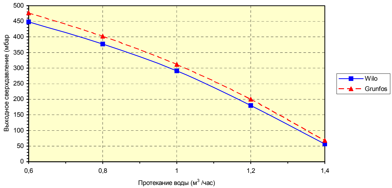
Присоединительное сверхдавление THERM 20 и 28 CX
