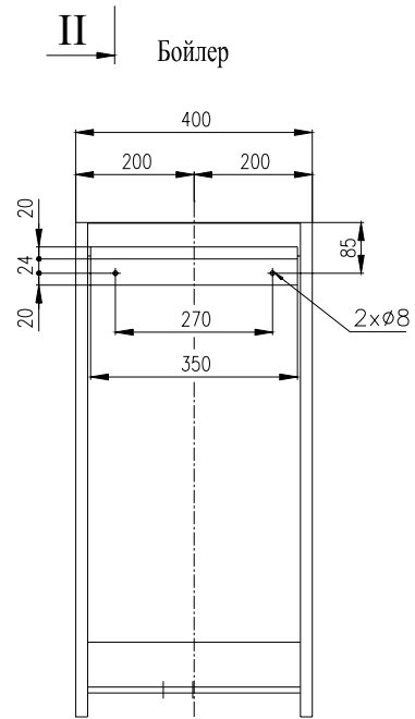
II | Разрез по II-II
